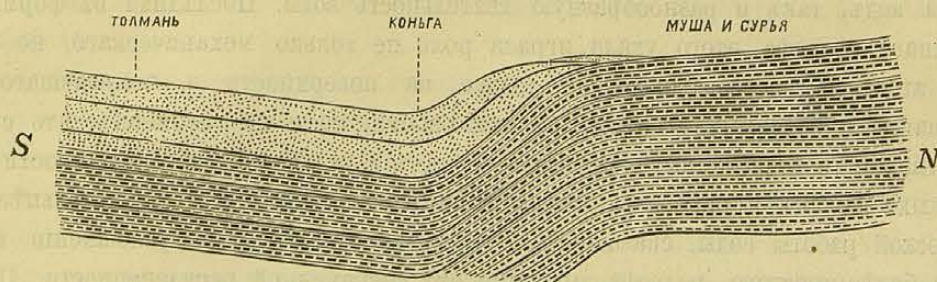
Продольный разръзъ пониженной части Вятскаго увала.
