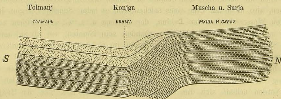
Längsdurchschnitt durch die Senkung des Wjatkaschen Rückens.
