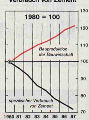
Bauproduktion und Verbrauch von Zement
