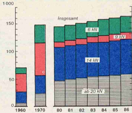
Traktorenbestand nach der Zugkraft
