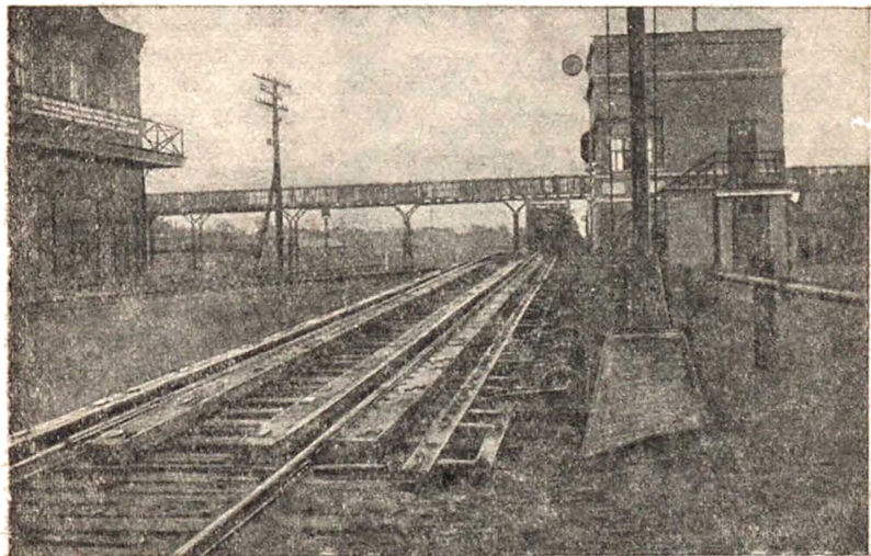
Механизированная горка
