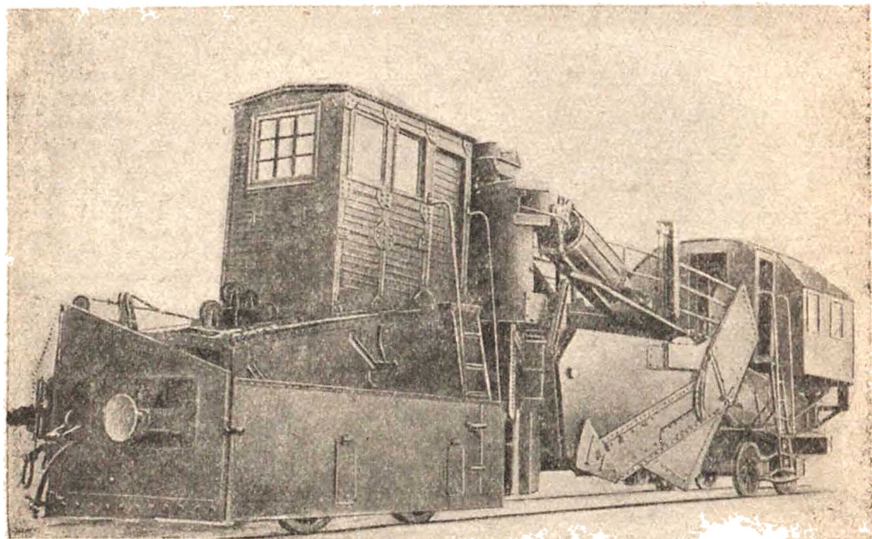
Путевой струг
