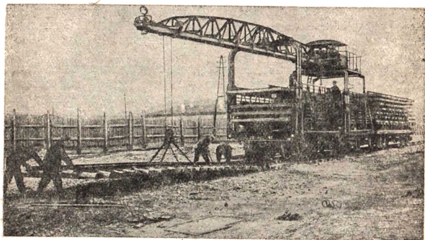
Путеукладчик Платова
