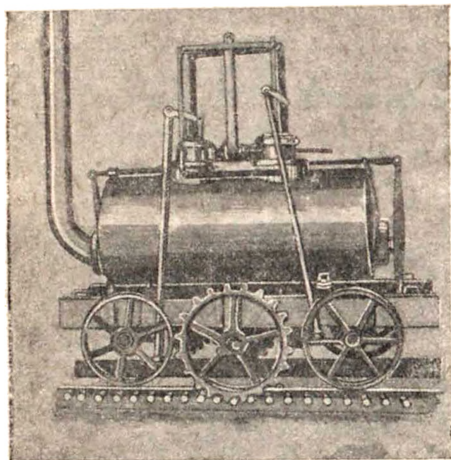
Паровоз Бленкинсопа
