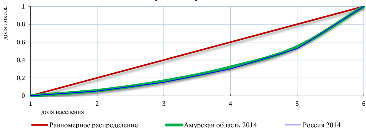
Кривая Лоренца
