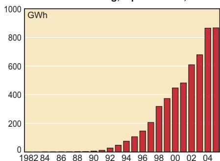
Vindkraftens utveckling, elproduktion, GWh
