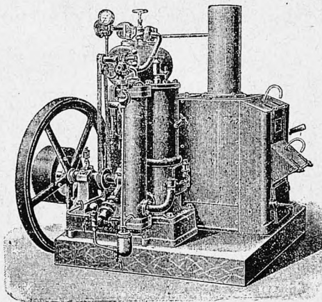
Экономическіе паровые двигатели. (GAGGENAUER DAMPF-SPARMOTOR). отъ 1 до 30 лощ. силъ.
