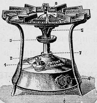
Керосино - газовая кухня
