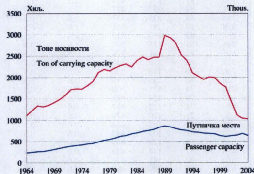
Граф. 15.4. ПРЕВОЗНИ КАПАЦИТЕТИ CARRYING CAPACITY
