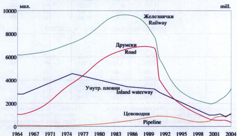
Граф. 15.6. ТОНСКИ КИЛОМЕТРИ ПО ВРСТАМА САОБРАЋАЈА TON-KILOMETRES BY TRANSPORT TYPE
