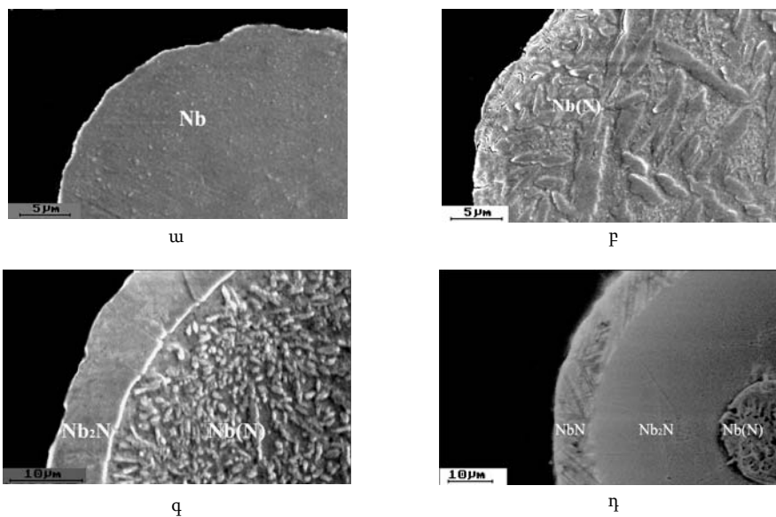
Նկ. 1: Նիոբիումի լարի ընդլայնական հատույթի ԼԷՍ-պատկերները. ա) էլային լար; բ) T = 2100^{\circ}\text{C} , P_{\text{N}_2} = 20 Տորր, t = 4 ւ: գ) T = 2100^{\circ}\text{C} , P_{\text{N}_2} = 100 Տորր, t = 0,5 ւ; դ) T = 2100^{\circ}\text{C} , P_{\text{N}_2} = 300 Տորր, t = 5 ւ:
