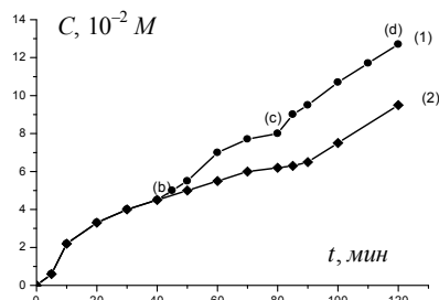
Рис. 1. Кинетические кривые полимеризации АК: кр. 1 (•) – водный раствор; кр. 2 (■) – двухфазная система вода–бензол (2:1).
