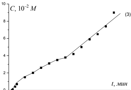
Рис. 2. Кинетическая кривая полимеризации АК в двухфазной системе вода–жир (1:1).
