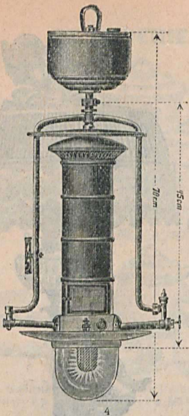
4. Инвертный Керосинно-налильный фонарь для внутреннего освещения, сила света 200 свѣчей; специально для фабрикъ, складовъ, ресторановъ и проч. 28 р. При каждомъ фонарь высылается руководство.
