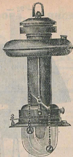
3. Клара—Спирто-налильный фонарь для наружного освѣщенія, сила свѣта 80 свѣчей, для дворовъ, фабрикъ, имѣній и складовъ—15 р.
