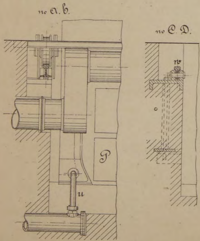
Черт. 233.
