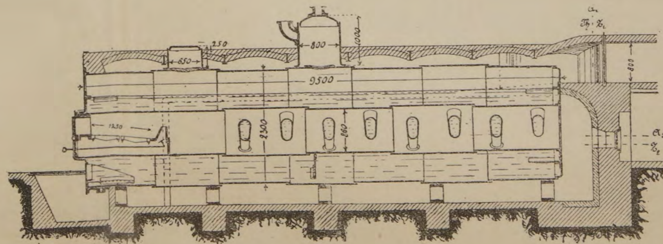
Черт. 140.
