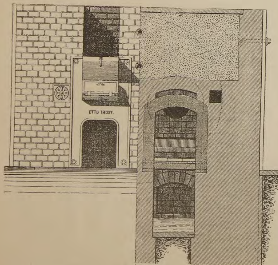
Черт. 43.
