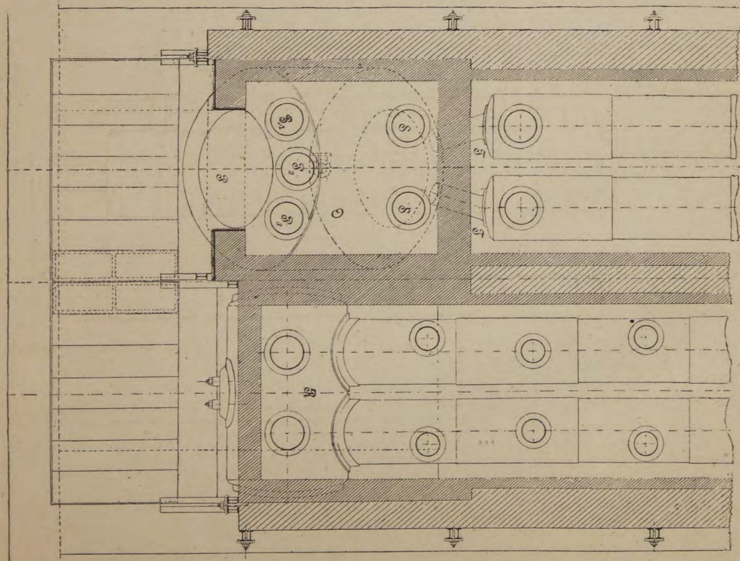
Плано во разрезе по CD.
