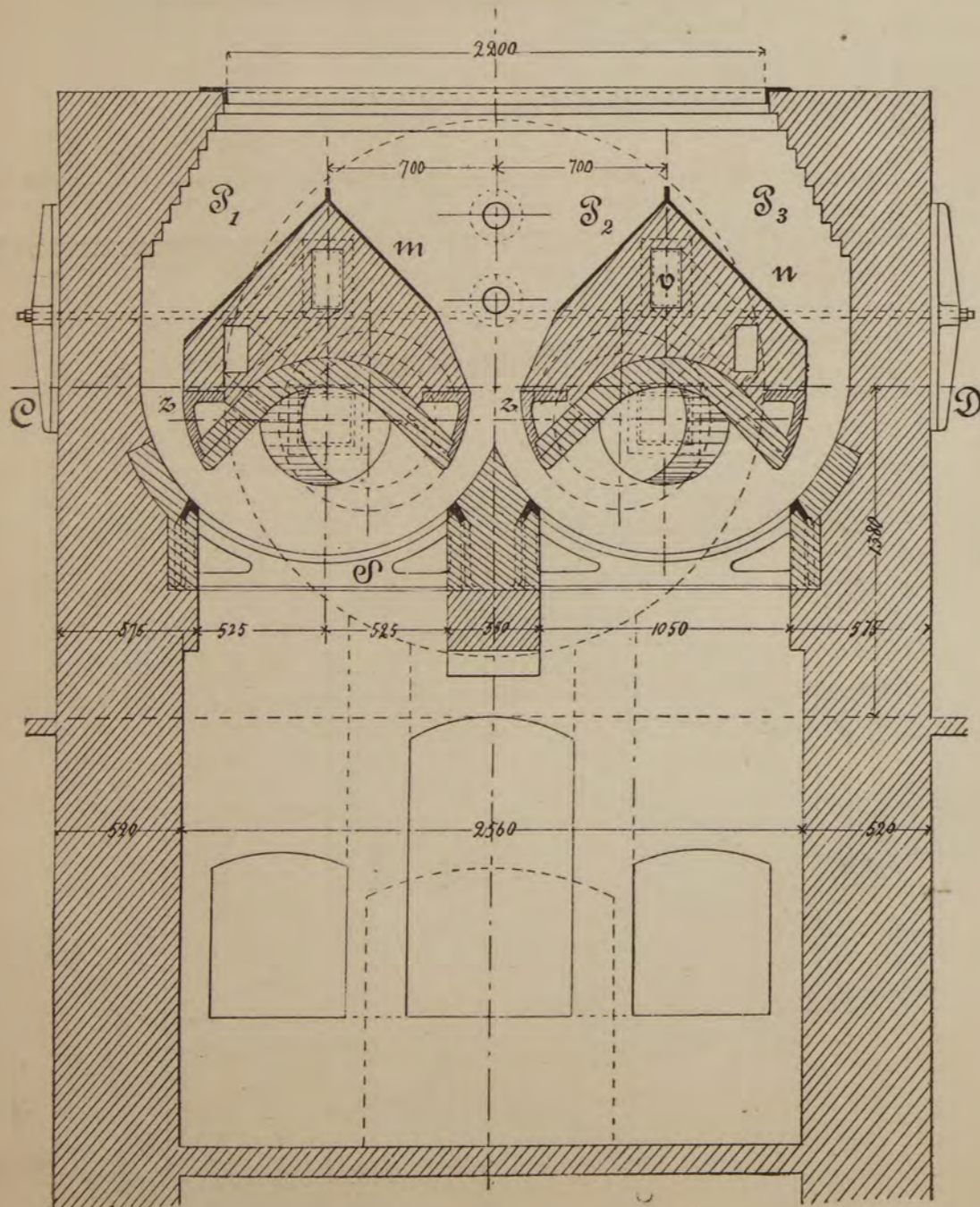
Черт. 64.
