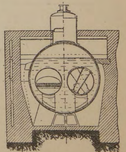
Черт. 141.
