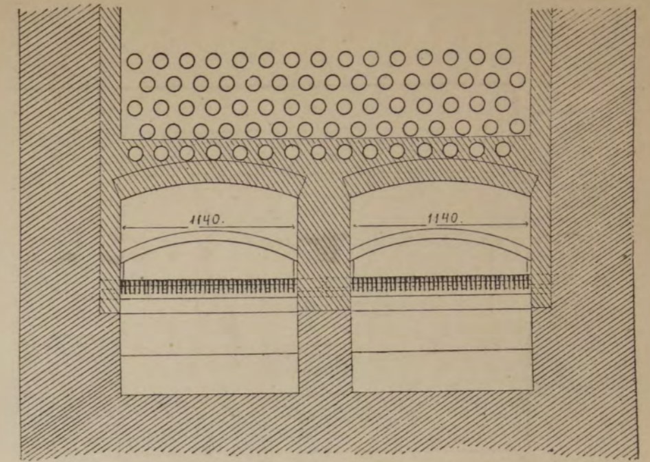
Черт. 138.
