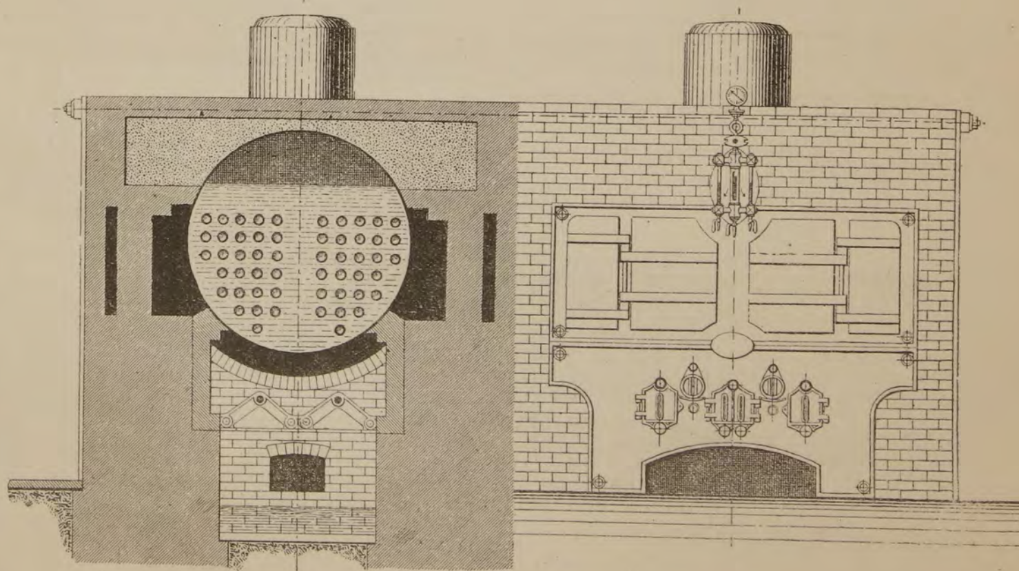
Черт. 56.
