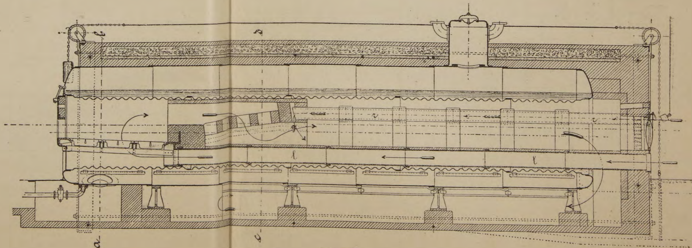
Черт. 67.
