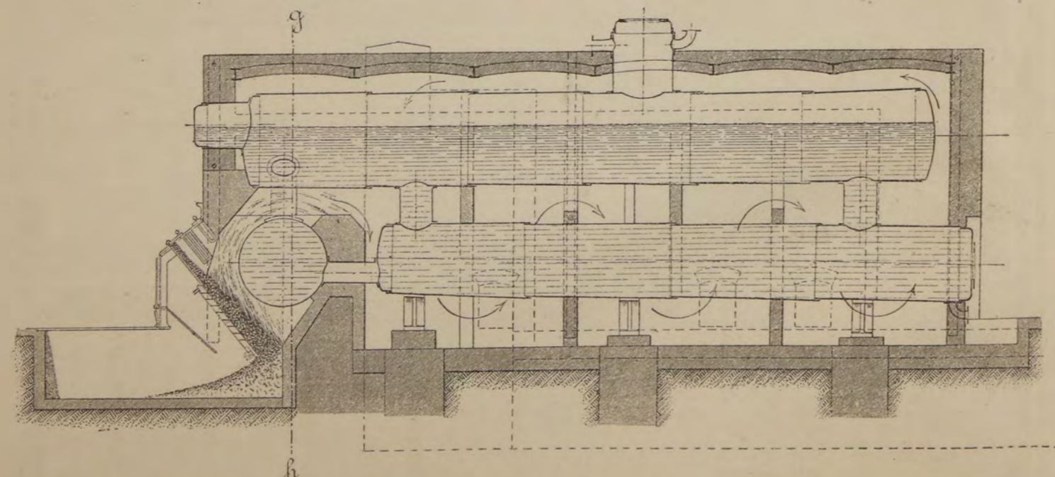
Черт. 120.
