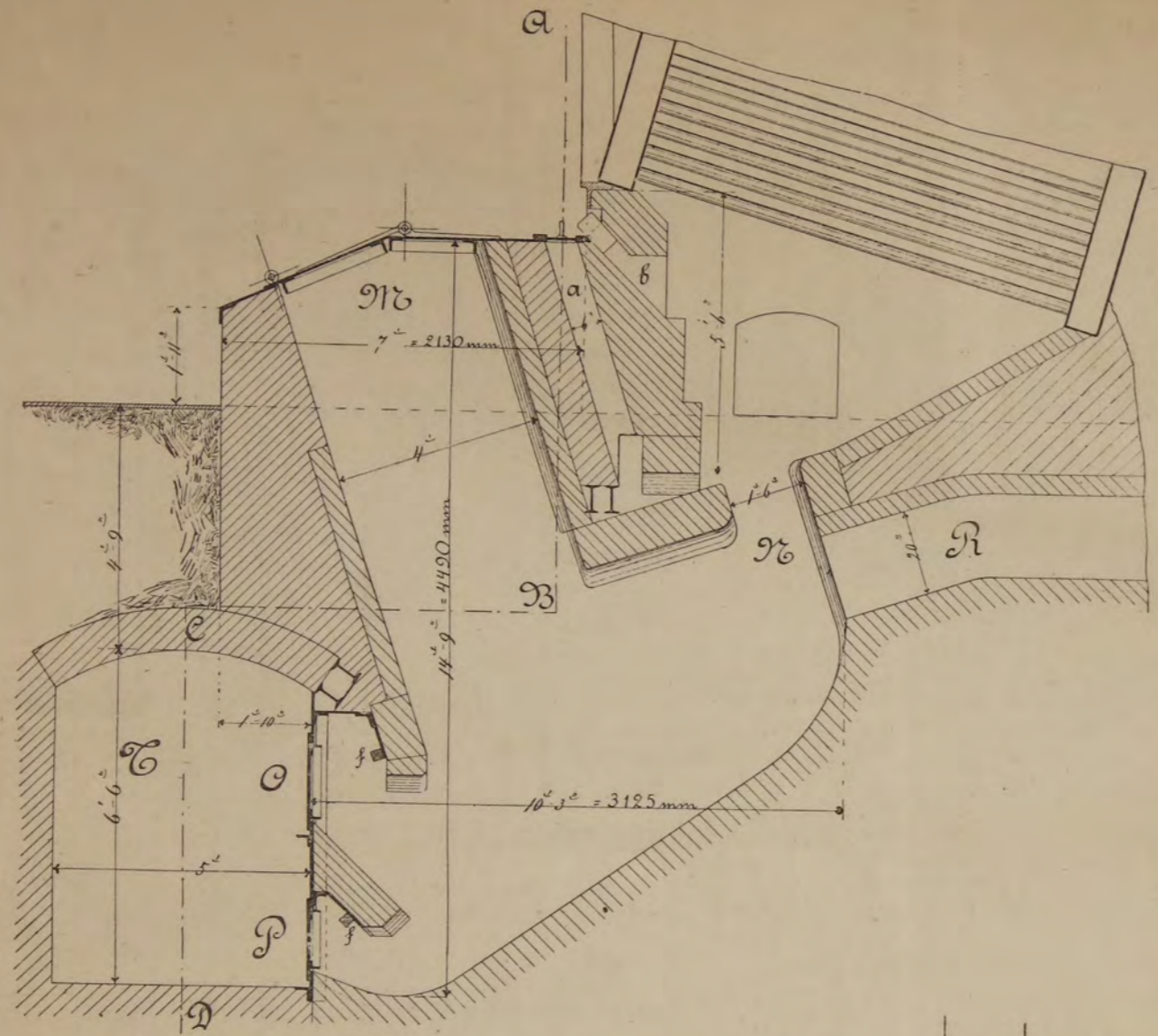
Черт. 239.
