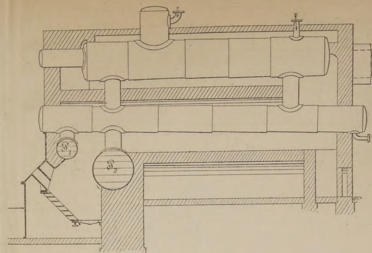
Черт. 117.
