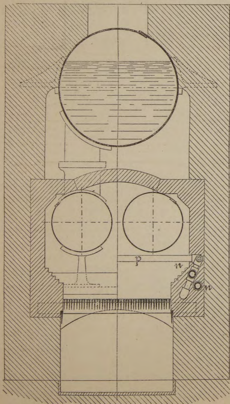
Черт. 151.
