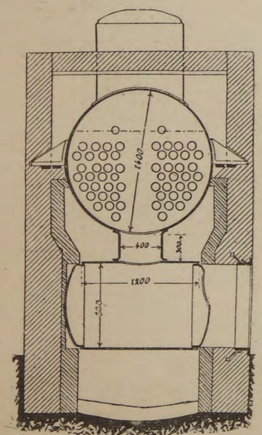
Черт. 116.
