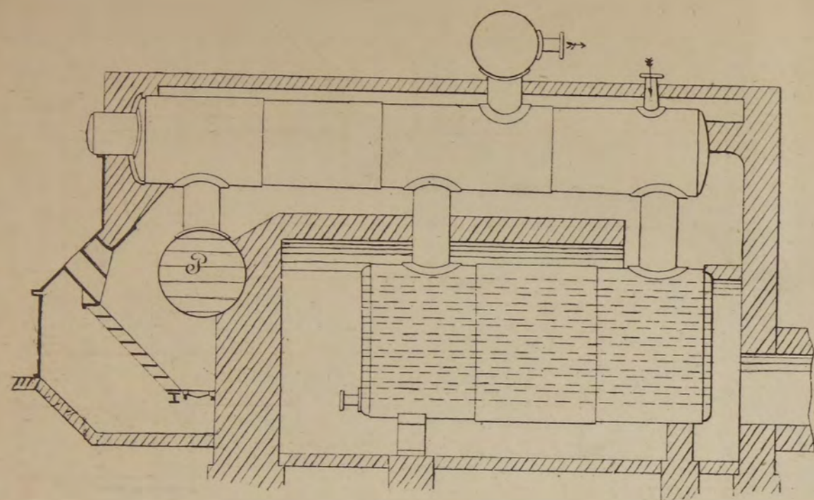
Черт. 114.
