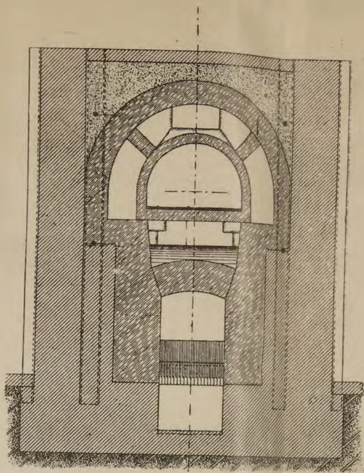
Черт. 47.
