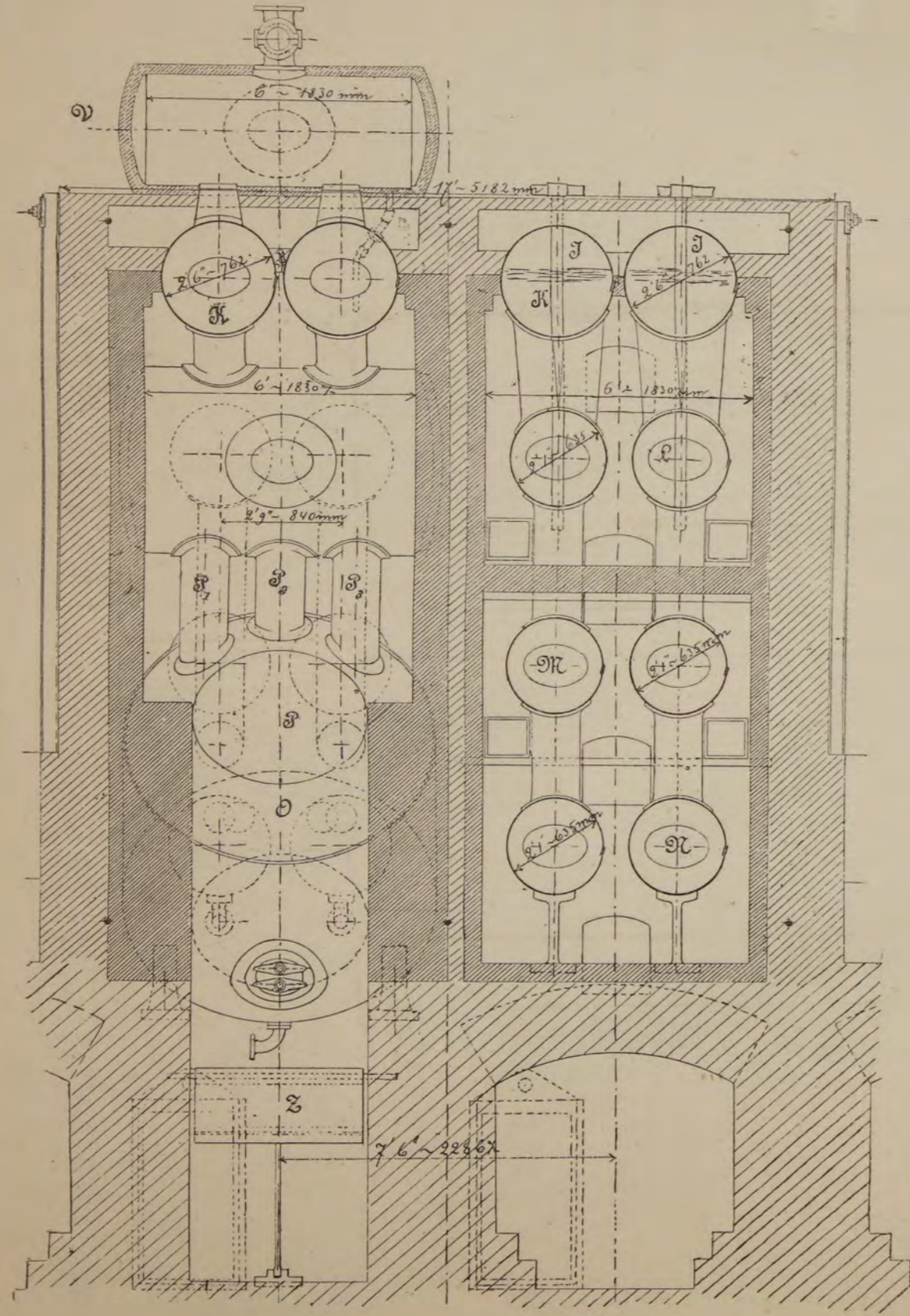
Черт. 101.
