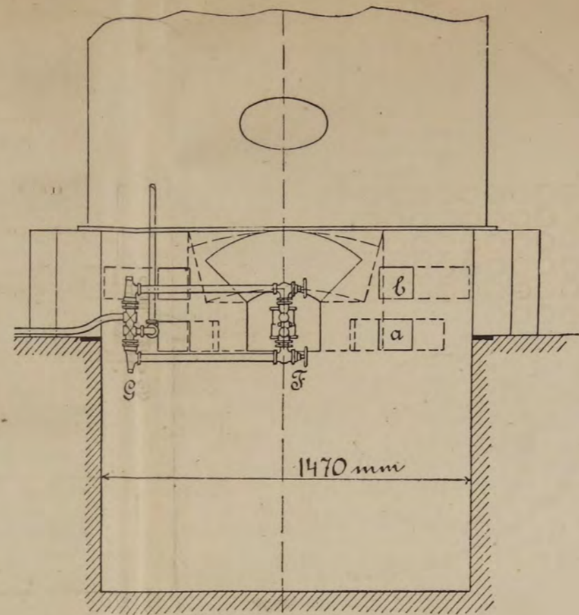
Черт. 201.
