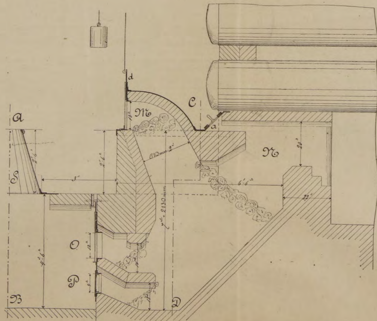
Черт. 236.
