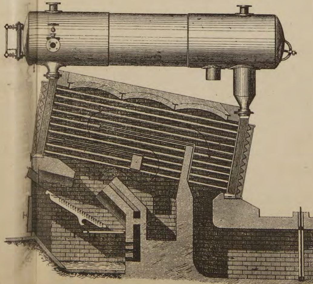
Черт. 39.
