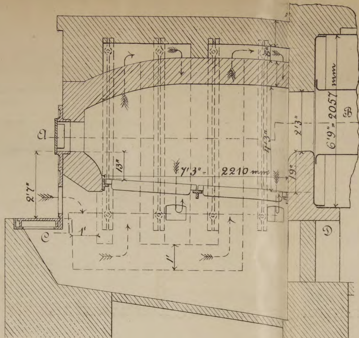
Черт. 59.
