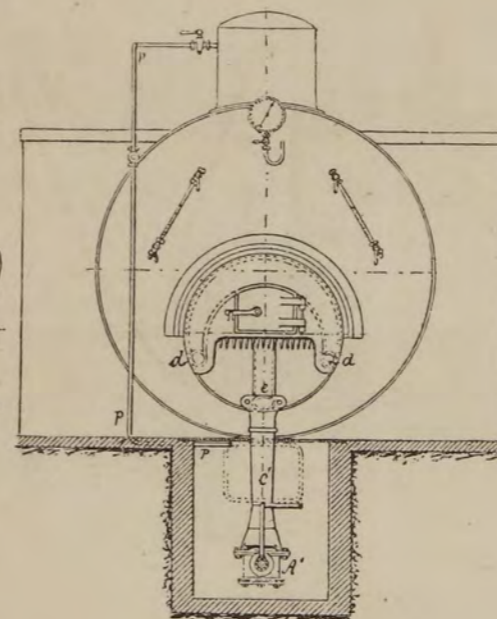
Черт. 165.
