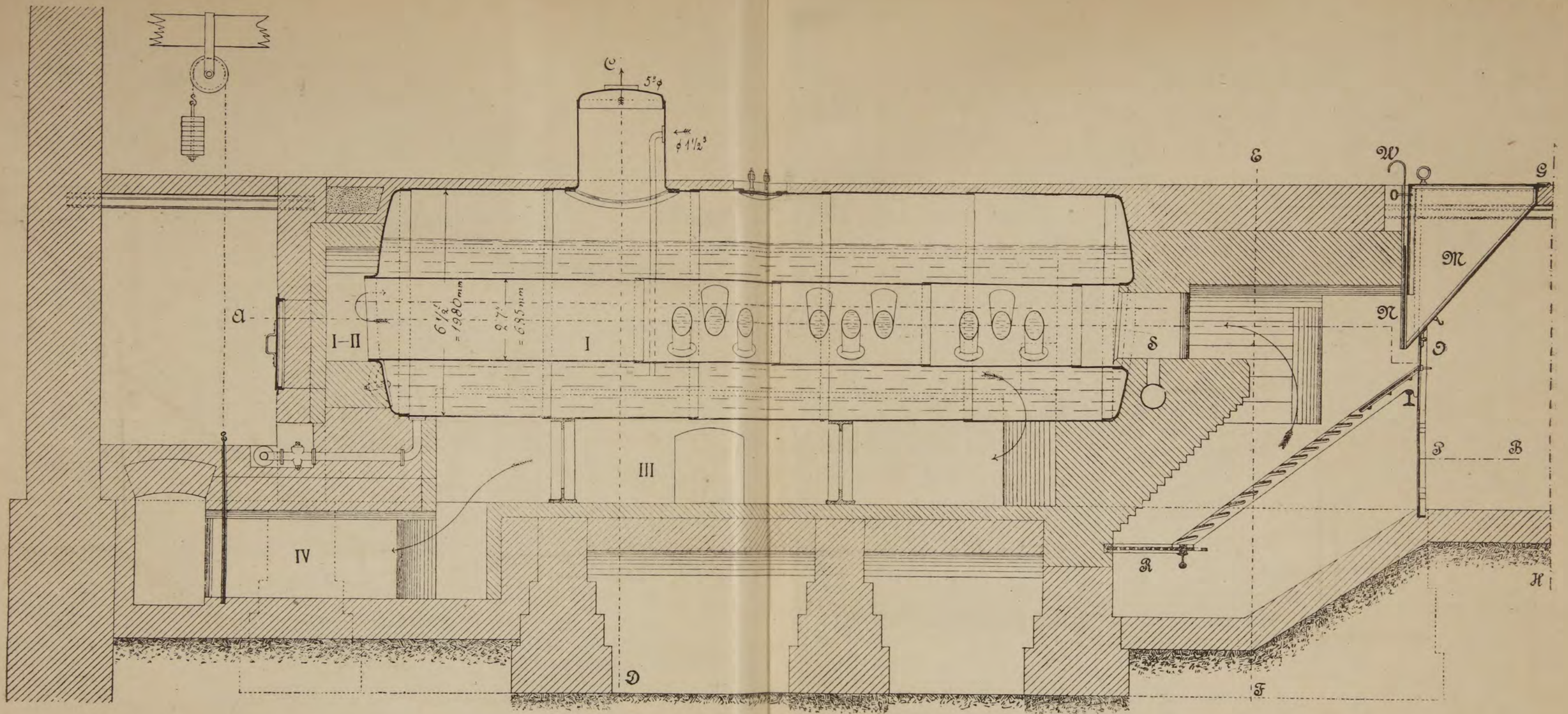
Черт. 35.
