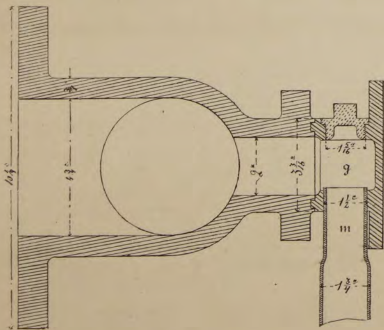
Черт. 19.
