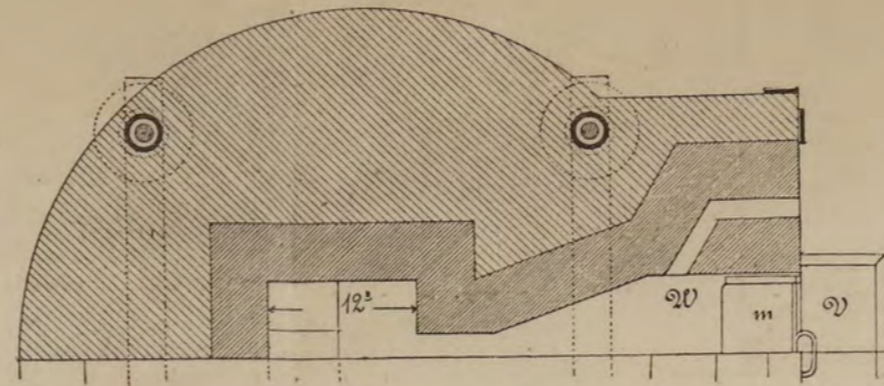
Черт. 181.
