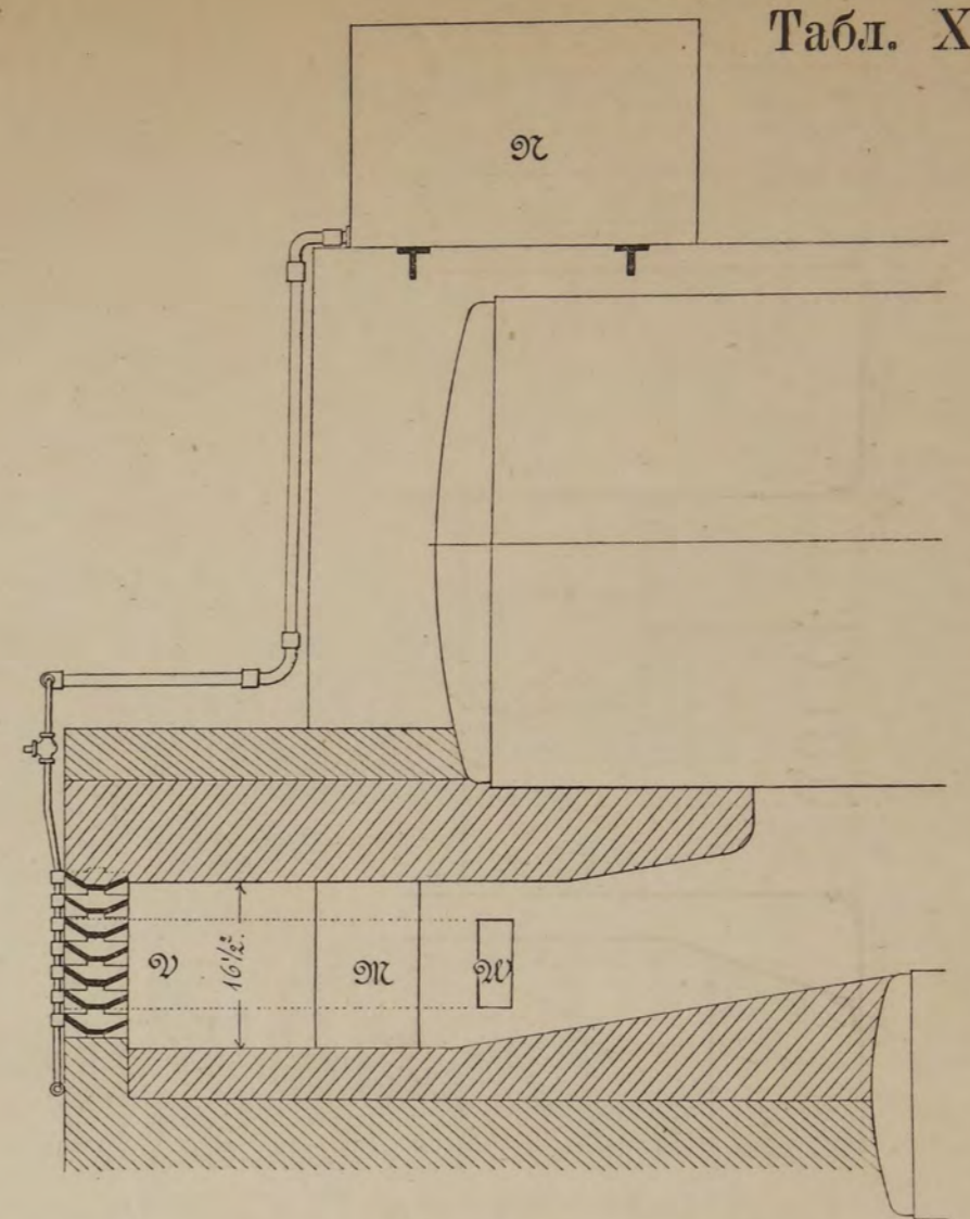
Черт. 177.
