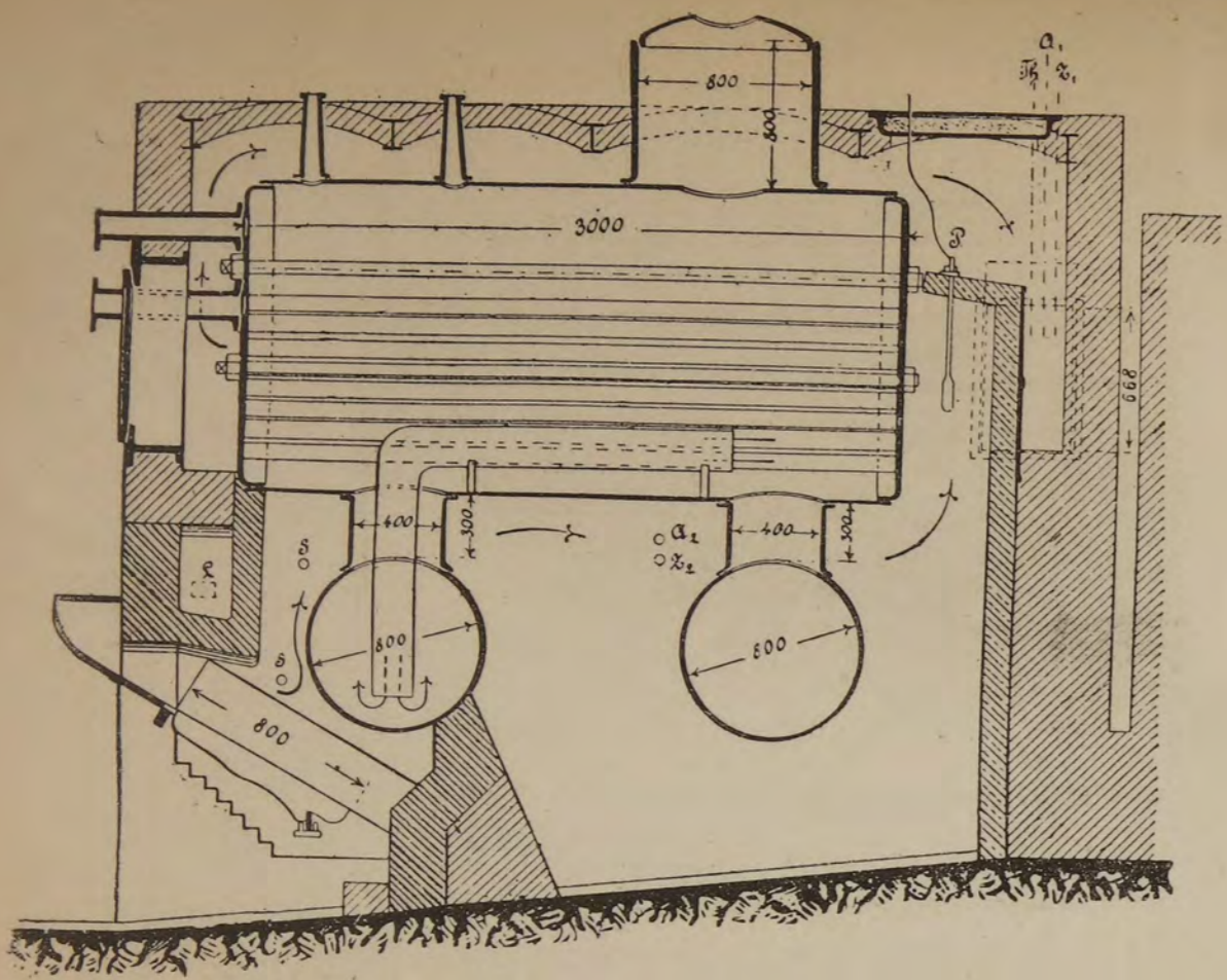
Черт. 115.
