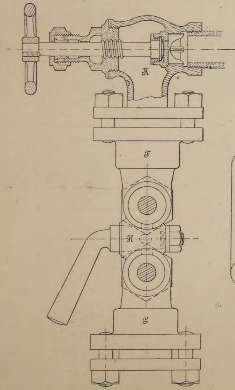
Черт. 185.
