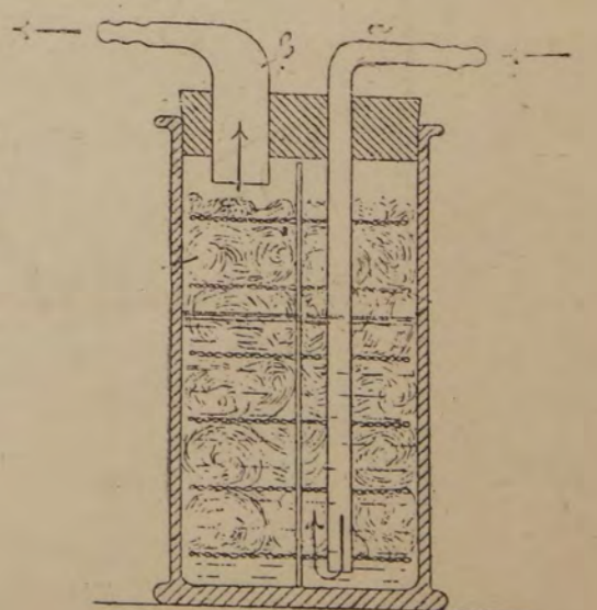
Черт. 245.
