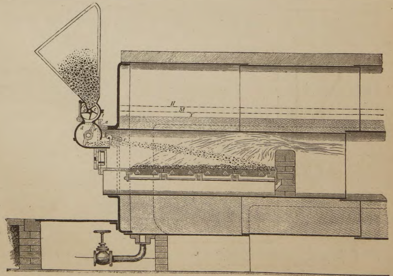
Черт. 73.
