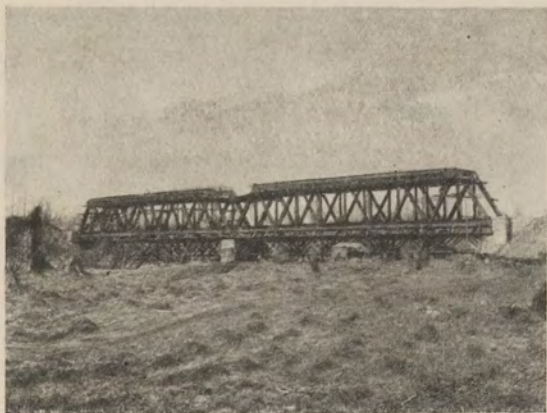
Рис. 12. Видъ моста черезъ рѣку Верхне-Олонгро по окончаніи работъ установкѣ и сборки фермъ. Верста 171-я. Пикетъ 162-22,50.
