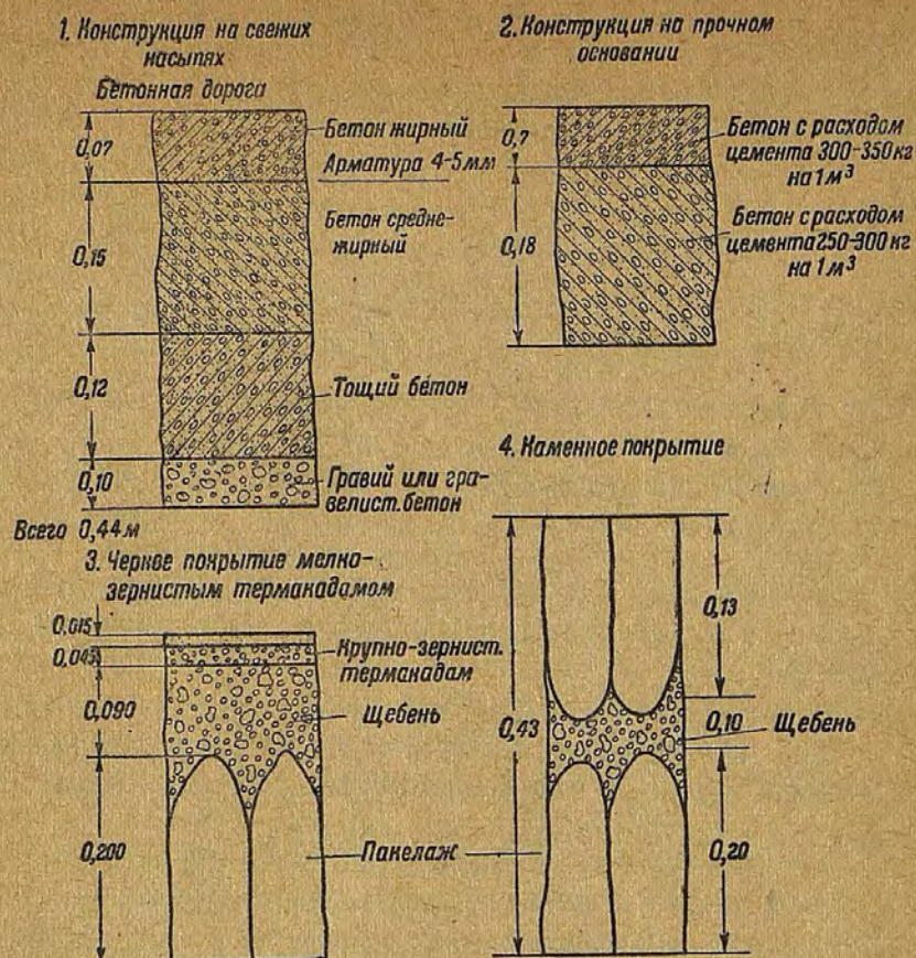
Схема 19. Типы покрытий германских автострад.
