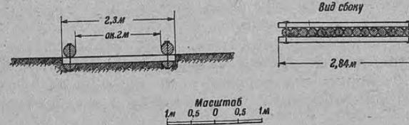
Система инженера Ильина (звено)
