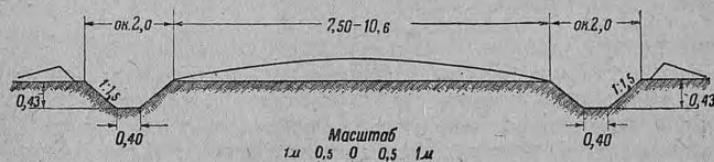
Тип 2-й — планировка с устройством полотна
