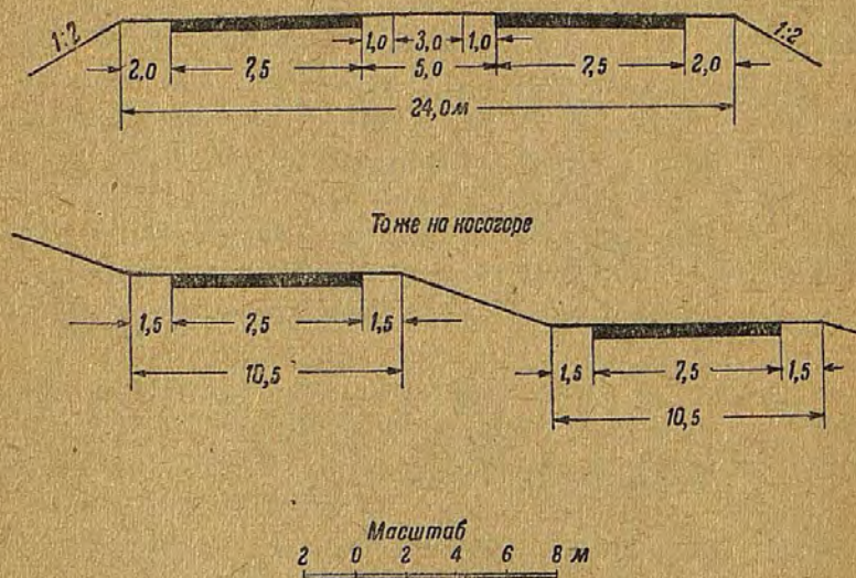
Схема 20. Германские автострады (поперечный профиль). Каждая полоса шириной по 7,5 м делится на полосы движения и обгона, шириной по 3,75 м каждая. В бетонных дорогах границей между ними служит шов. Промежуток между полосами засаживается на 3 м деревьями. Обочины с обеих внешних сторон наполовину укрепляются промасливанием.
